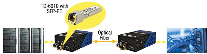
FOI-6010 or FOI-6012 Fiber Optic Isolator Transceiver Workbox
