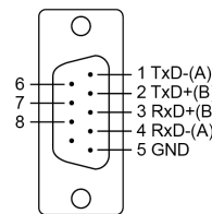
RS-422/RS-485-4w
