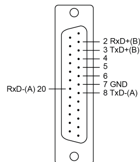
RS-422/RS-485-4w
