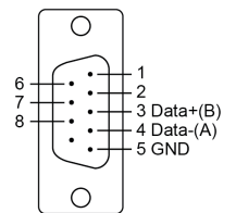
RS-485-2w
