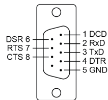
RS-232
