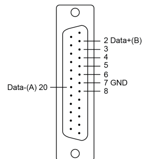
RS-485-2w
