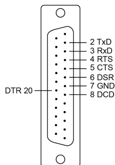
RS-232
